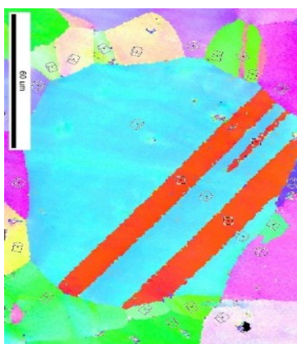
Abb. 3: EBSD (IPF-coloring), Schichtoberfläche
