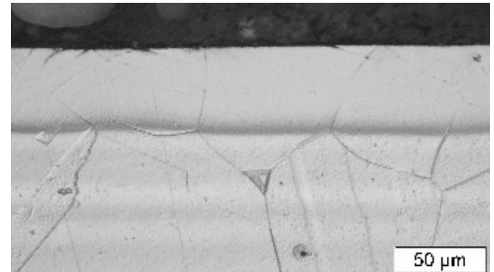
Abb. 1: Querschliff geätzt, Schicht
