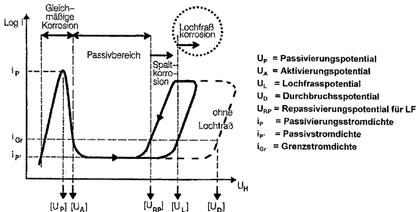
Abbildung 1: schematische Darstellung einer Stromdichte-Potentialkurve von einem passiven Metall
